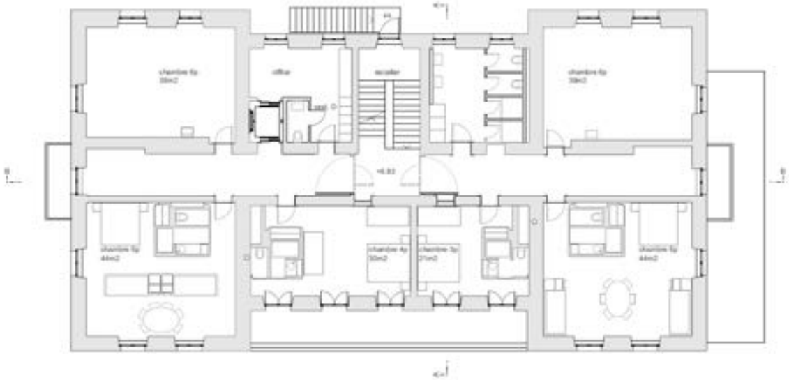
GayMennel, architectes epb, dlight Avenue de l'Industrie 8 CH-1870 Monthey Tel +41 24 475 70 80 mail@gaymennel.com Grand Hôtel du Cervin à St-Luc plan 2ème étage 1/100, 12.12.2017
