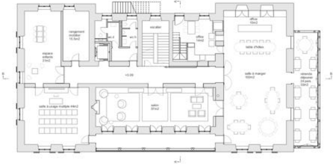
GayMennel, architectes epb, dlight Avenue de l'Industrie 8 CH-1870 Monthey Tel +41 24 475 70 80 mail@gaymennel.com Grand Hôtel du Cervin à St-Luc plan 1er étage 1/100, 12.12.2017
